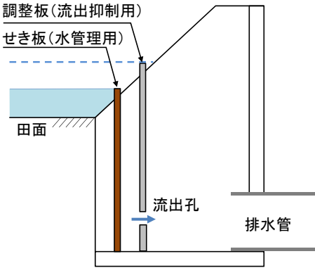
排水柵の構造
